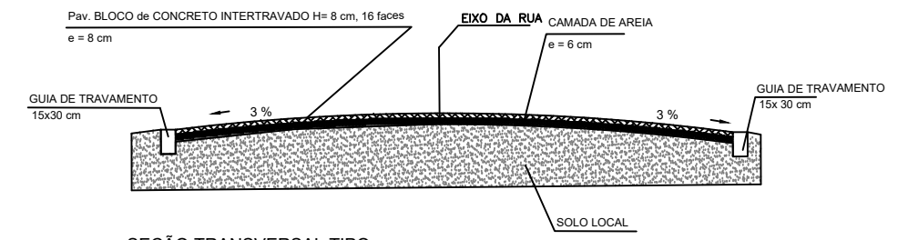
SEÇÃO TRANSVERSAL TIPO Sem escala
